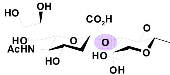
\alpha 2,3 Sialic acid
